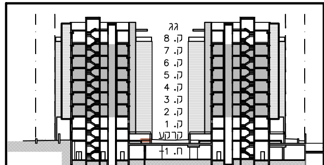
חתך סכמטי
